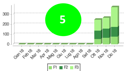
Andamento Energia Attiva (kWh)
